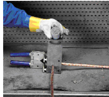
STEP 3: Pour weld metal into mold.
